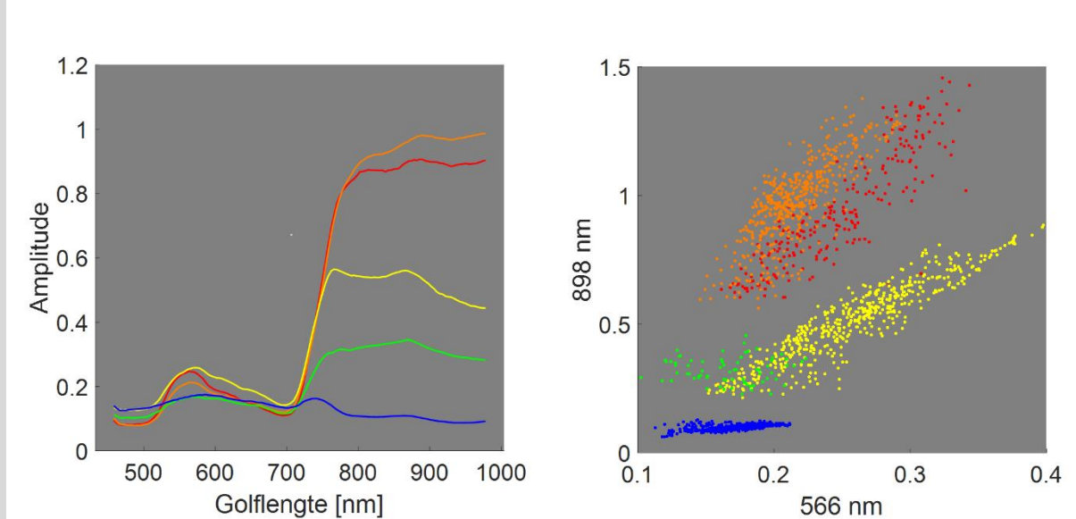
Afbeelding 2. Voorbeeld van de mogelijkheden van de Cubert S185 Firefly SE hyperspectrale camera om verschillende vegetatie te classificeren. (a) Zwart-witbeeld (1000x1000 pixels), (b) selectie van verschillende klassen (50x50 pixels), (c) mediaanspectra van de verschillende groepen en (d) geïdentificeerde klassen, geplot voor de pixelwaarden van 898nm tegenover 566 nm. NB: de rode groep bestaat uit gemaide oevervegetatie
